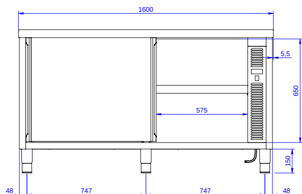
Alzado
